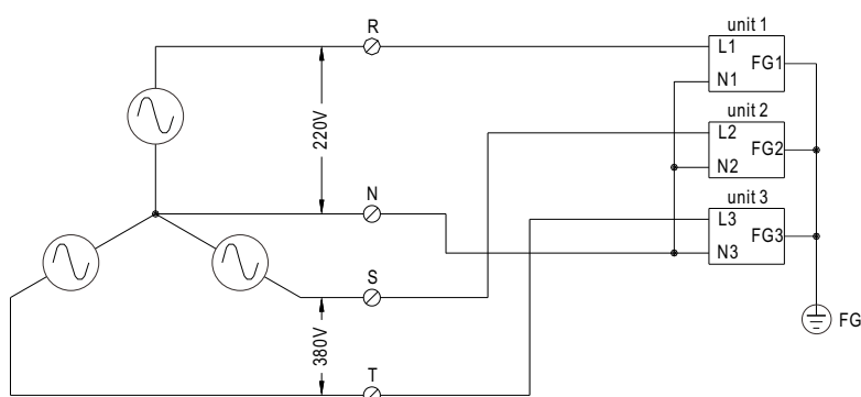
※FIG. B: 3 \phi 4 wire 220/380VAC SYSTEM
