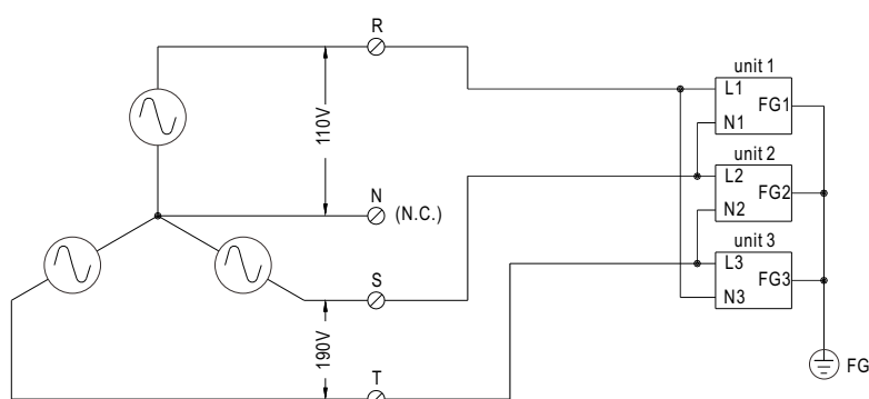
※FIG. C: 3 \phi 4 wire 190/110VAC SYSTEM
