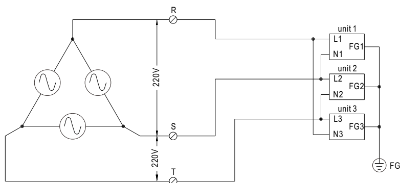
※FIG. A: 3 \phi 3 wire 220VAC SYSTEM
